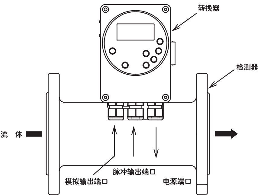
图 1-1 流量计的流量测量系统的图示。
