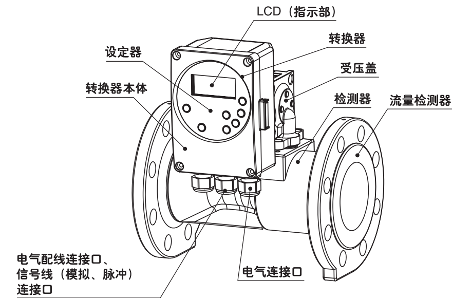
图 1-3 流量计的结构
