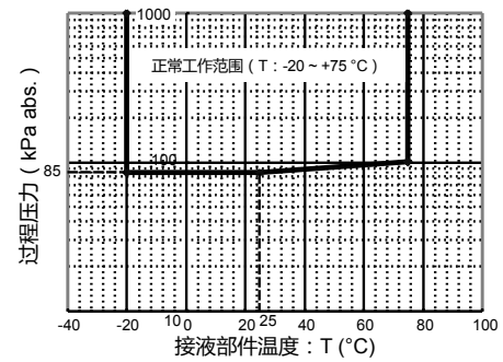
图 3. 型号 PTG_G 和氟油组合的最小工作压力。
