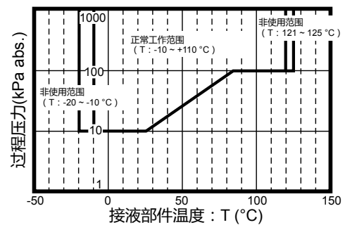
图 7. 型号 PTG_S 的最小工作压力。 对于 PTG_S 防脉动型 (-J), 正常工作温度范围为 10 ~ 45°C, 极限工作温度范围为 8 ~ 47°C。
