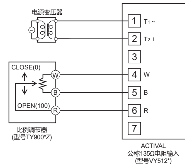
图16 与Neostat的连接例
