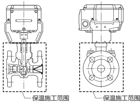
图6 保温施工
