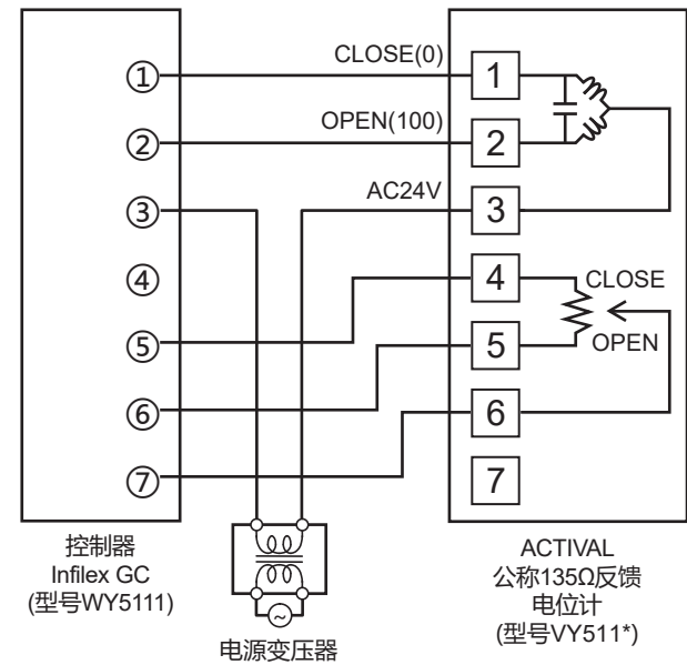
图15 与Inflex GC的连接例
